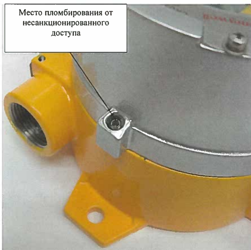
Рисунок 2 – Схема пломбирования газоанализаторов от несанкционированного доступа
